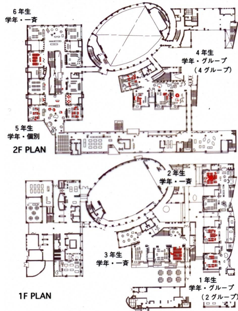
打瀬小学校 午前中の学習展開場面 1996/10/8
