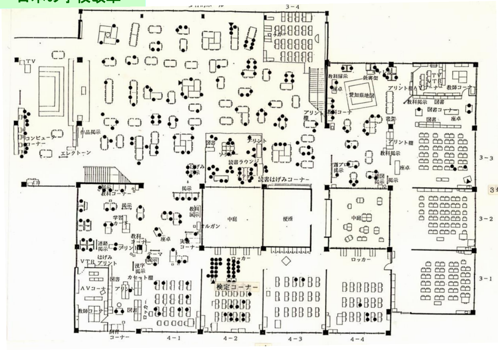
緒川小学校:愛知県東浦町:1979
