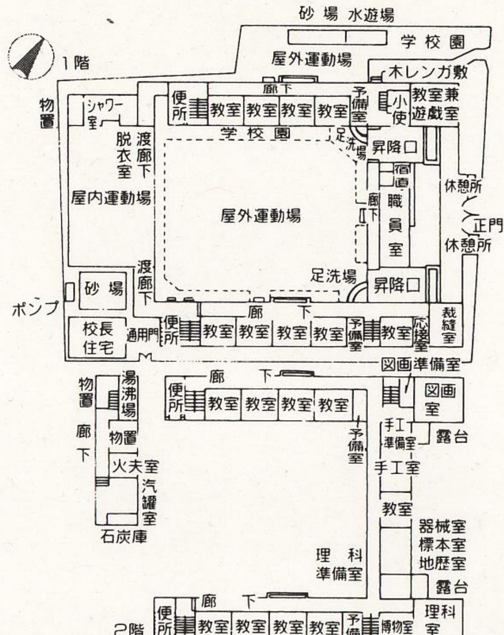
大正期のRC造校舎: 東京市番町小学校
