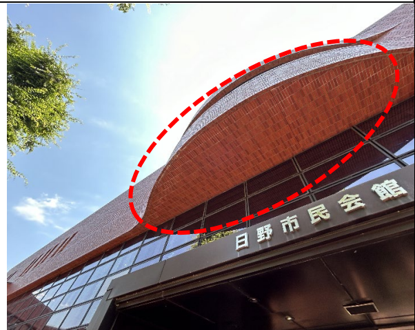
正面玄関バルコニー外壁(上裏) 白華現象
