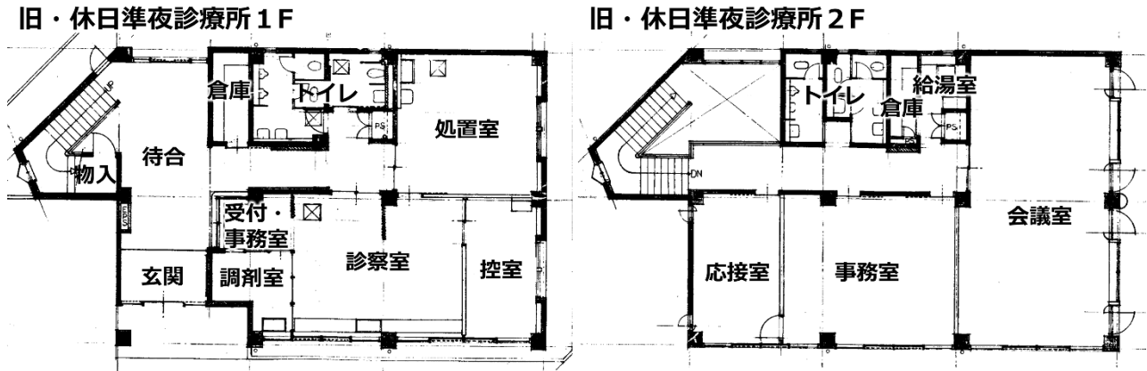
図 2.28 旧・休日準夜診療所の平面図 (※1) (日野市資料をもとに作成)
